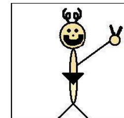
Helium
