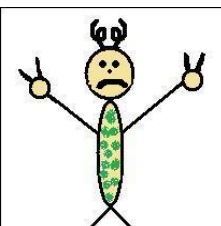
Beryllium
