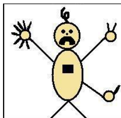
Sodium
